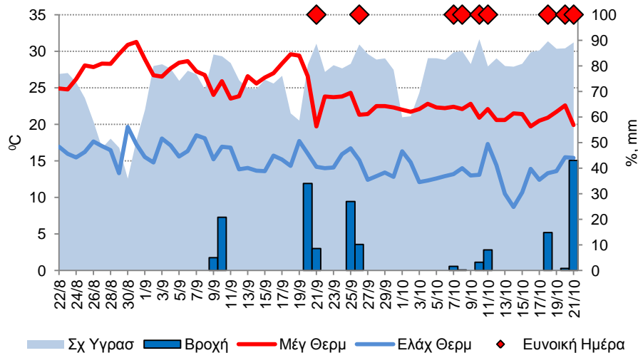
Διάγρ. 1 Μετεωρολογικός Σταθμός Σαγαϊκών Αχαΐας
